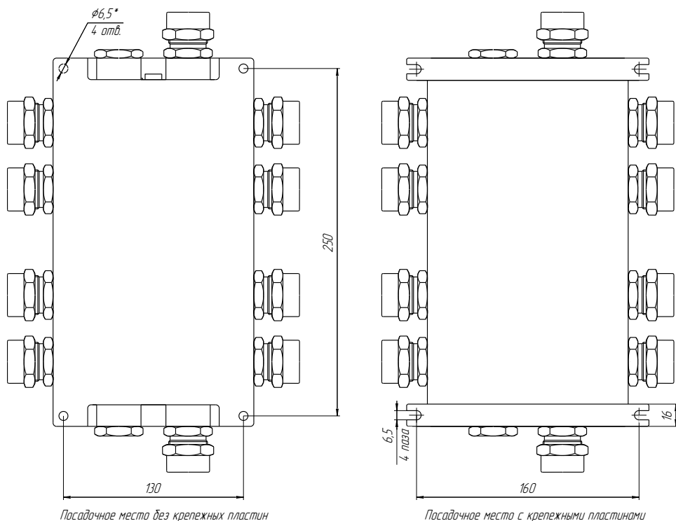
Рисунок 5 – Вариант крепления КС при помощи крепежных пластин
